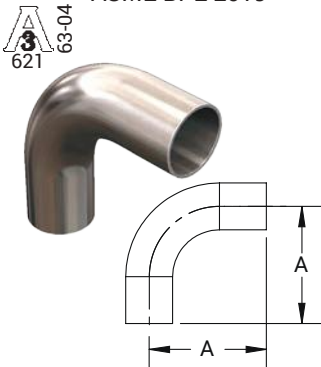
BPE Tabla DT-4.1.1-1 ASME BPE 2019
