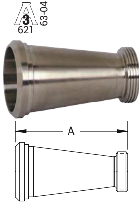
Reductor Concéntrico de Asiento Plano Biselado x Asiento Roscado Biselado - B3115F
