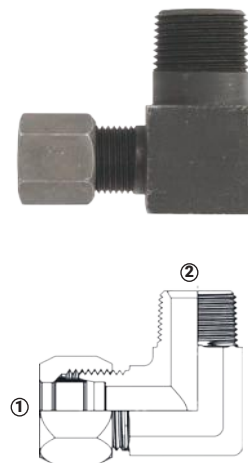
(1) Tubing Macho (2) Macho NPTF
