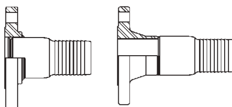
Brida con hombro cuadrado, slip-on con cara realzada
