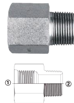
(1) Hembra SAE O-ring (2) Macho NPTF
