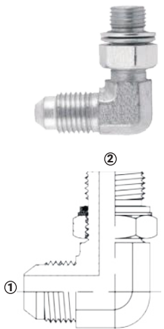
(1) Macho JIC (2) Macho métrico
